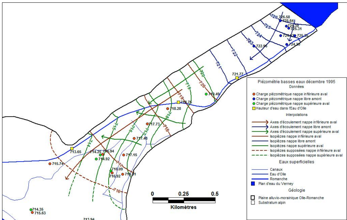
Carte piézométrique de la nappe de l'Eau d'Olle (données de décembre 1995)
