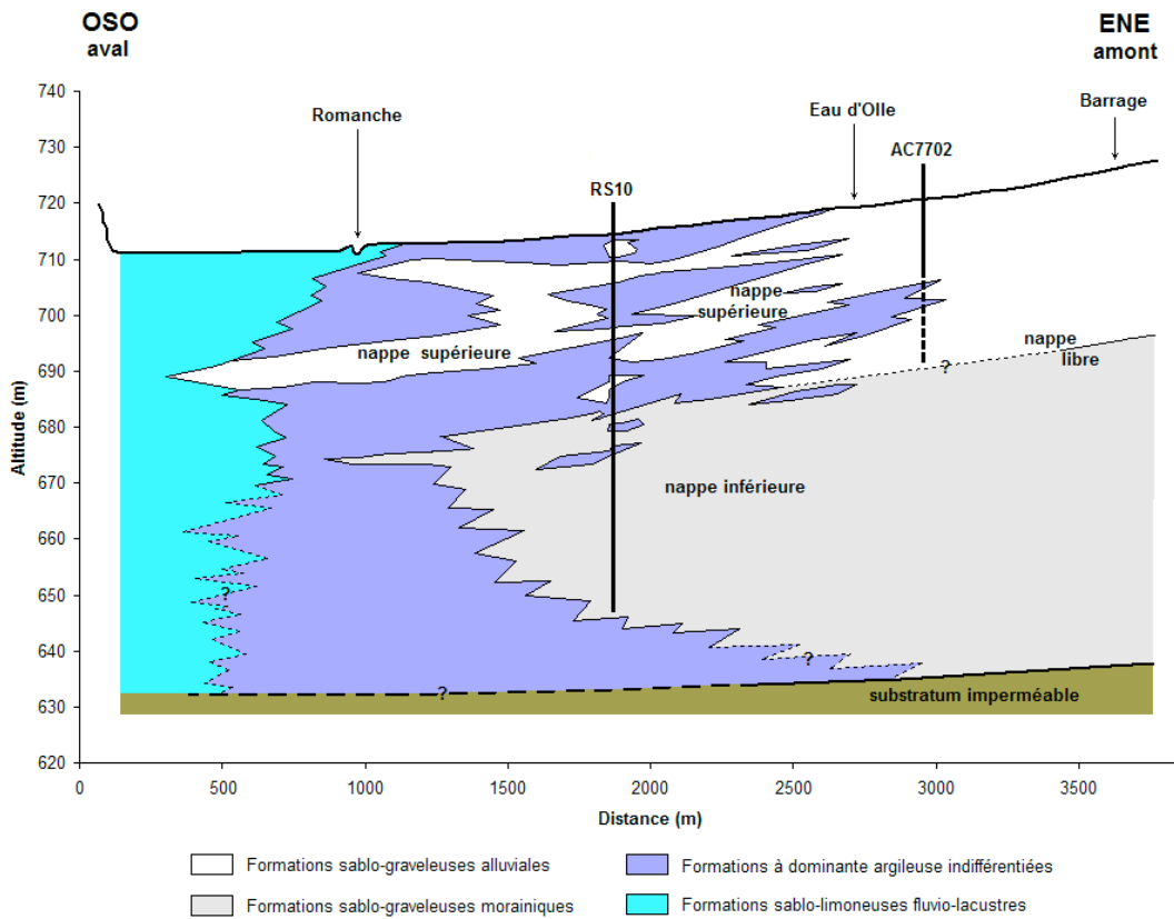
Coupe de l'aquifère de l'Eau d'Olle en aval du barrage
