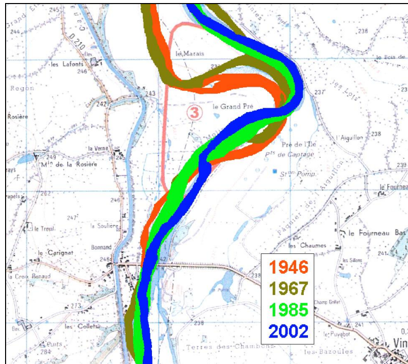
Divagation du lit de la Loire durant les 60 dernières années
