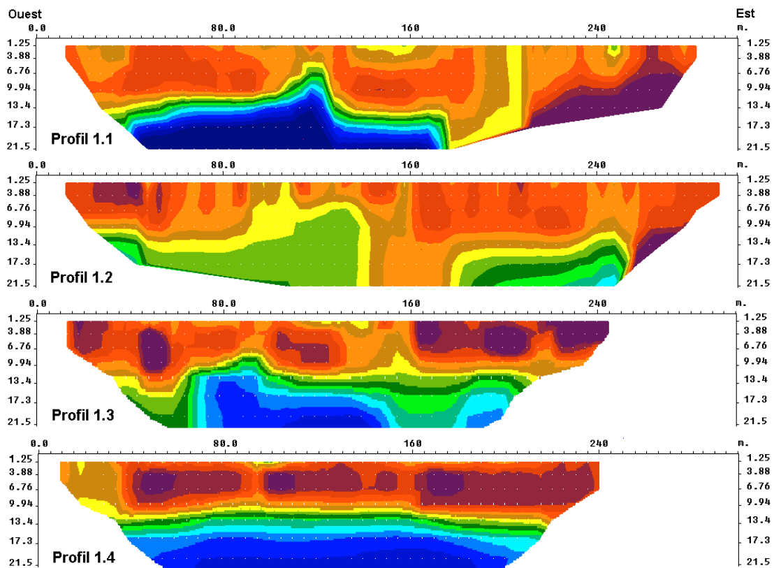
Investigation géophysique des matériaux alluviaux
